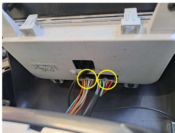
Irrota mittariston liittimet.
