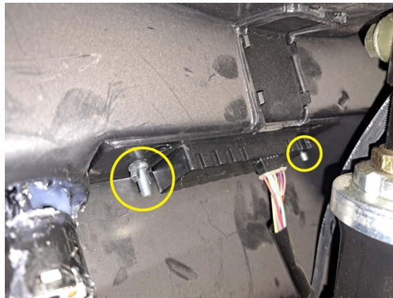
Irrota radion kiinnitys siipimutterit.
